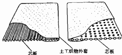
图 1 典型的塑料排水板(带)
