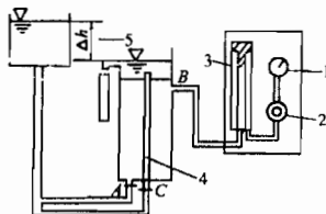
图 A.1 立式通水能力测试仪
