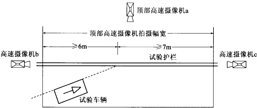
图5.7.5-1 高速摄像机布置示意图（适用于护栏标准段、护栏过渡段和中央分隔带开口护栏）
