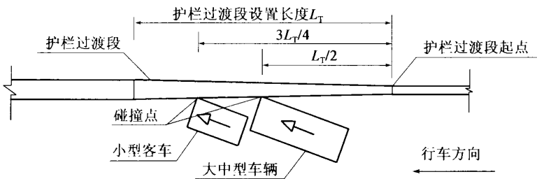
图 5.4.1-2 护栏过渡段的碰撞点位置
