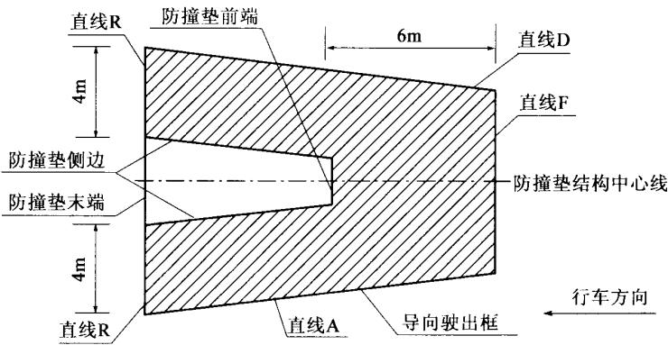
图 4.3.3-2 防撞垫的车辆轮迹导向驶出框
