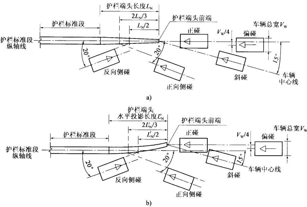
图4.2.1-2 护栏端头的碰撞类型
