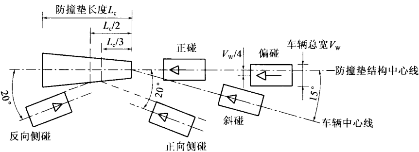
图 4.3.3-1 防撞垫的碰撞类型
