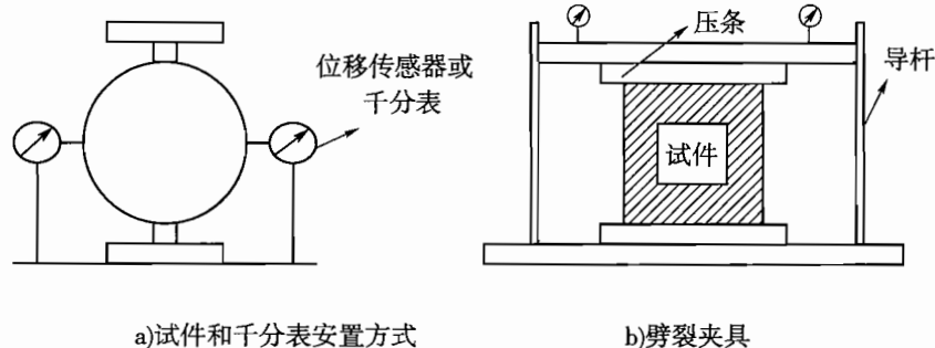
图 T 0852-1 劈裂回弹模量试验装置示意图
