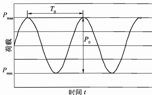
图 T 0856-1 疲劳试验荷载曲线示意图
