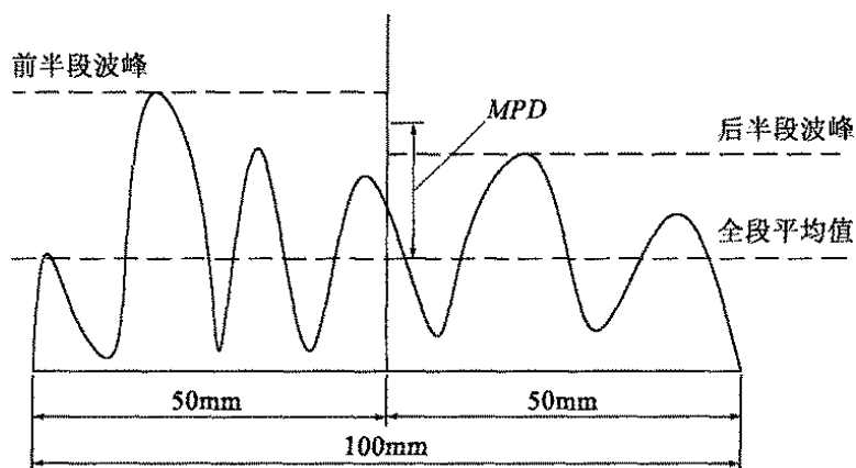
图 9-1 断面平均构造深度 MPD 计算方法
