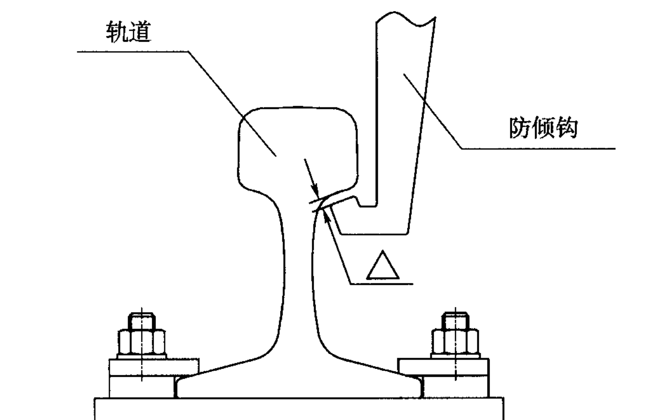
图 4.5.3-1 防倾保护装置与承载体之间的纵向间隙示意图
