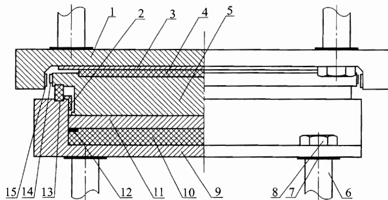
图6 减震型单向活动支座结构示意图
