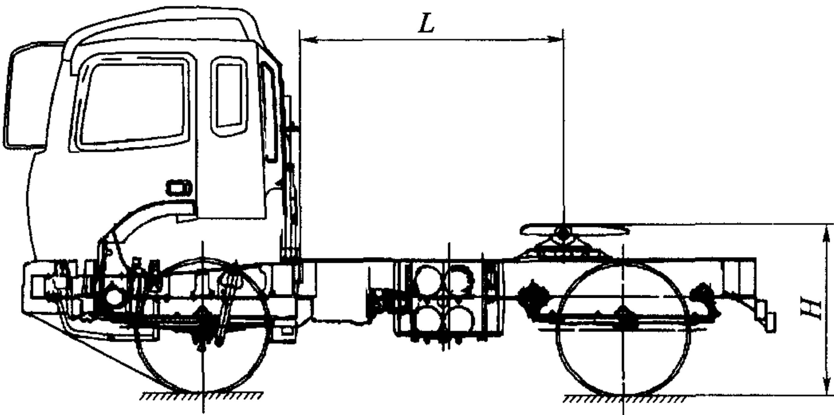
图 1 牵引车
