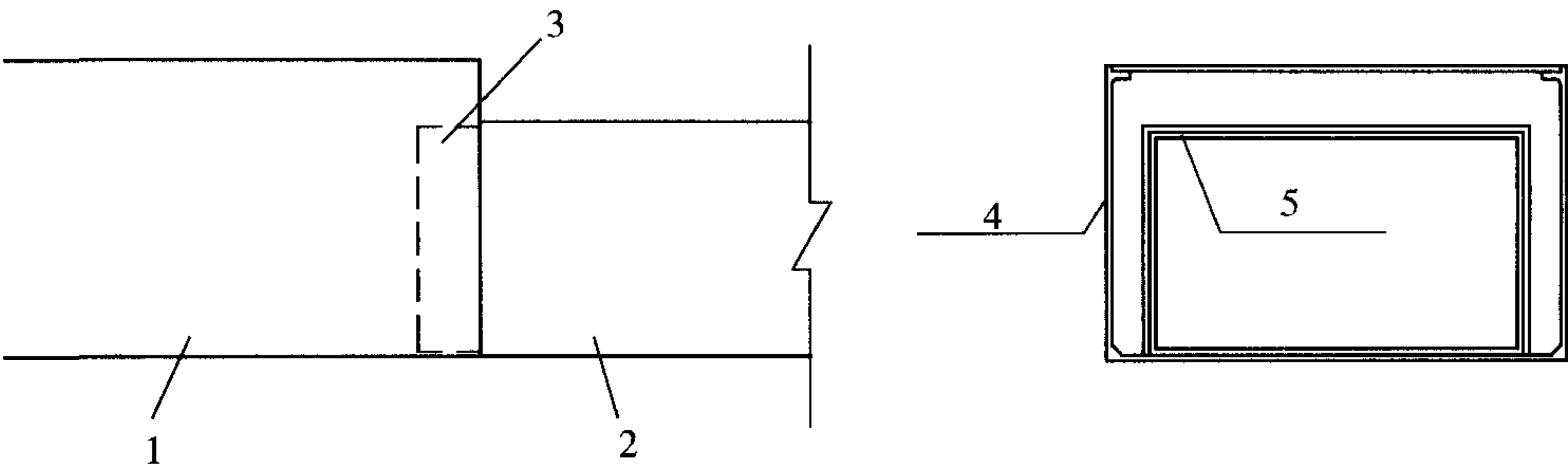
图 A.1 按照结构划分的管箱结构形式图
