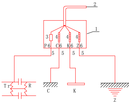
图 6.1.4 CD—I 型监测点接线盒示意图
