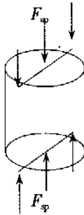
图 A. 2. 1 劈裂抗拉试验
