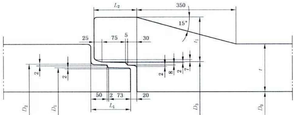
图 A.3 \phi 1\,350\sim\phi 1\,500 柔性接头 B 型承插口管接头
