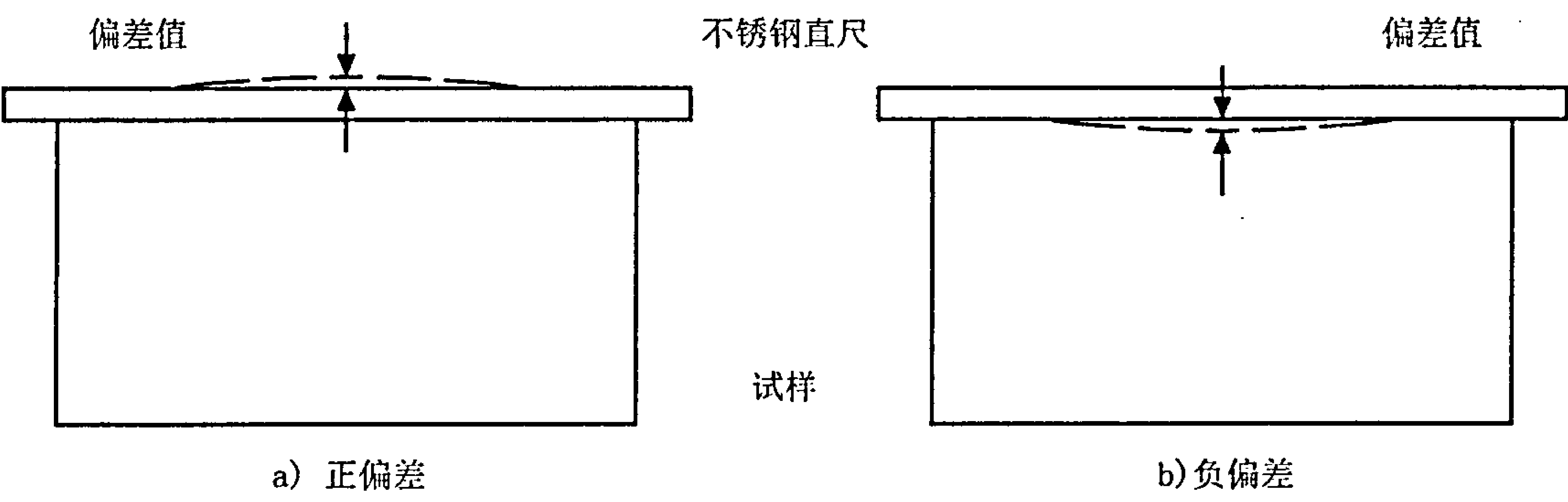
图A. 2 侧向弯曲测量示意图
