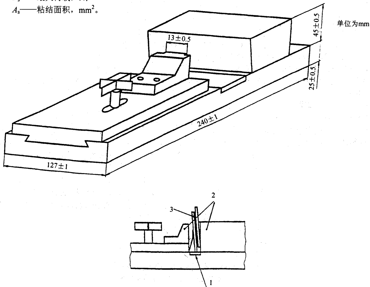
1—垫块；2—移动固定爪；3—试样。
