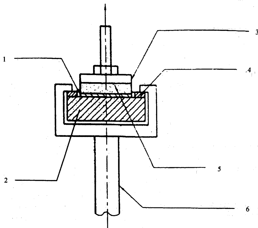
1—界面剂；2—70mm×70mm×20mm的砂浆试件；3—拉拔接头；4—垫块； 5—40mm×40mm×10mm的砂浆试件；6—拉伸试验夹具
