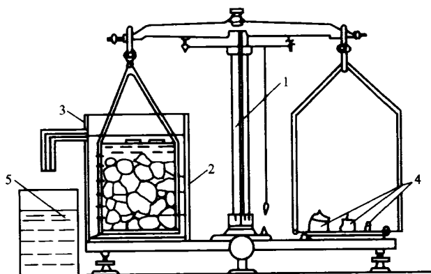
图 7.2.2 液体天平
