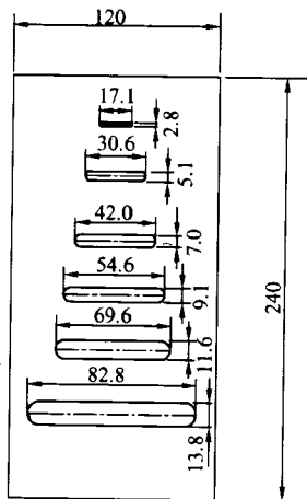
图 7.9.2-2 片状规 准仪 (单位: mm)
