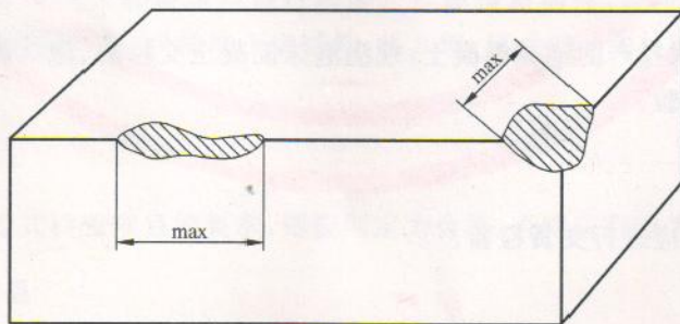
图 1 测量缺棱掉角示意图
