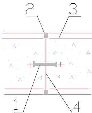
(a) 完全收缩缝
