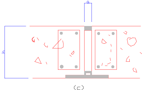
图 6.1.2 配筋形式
