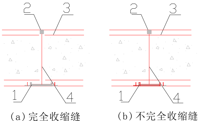
图 2.3.2—2 引发缝(外贴式止水带)
