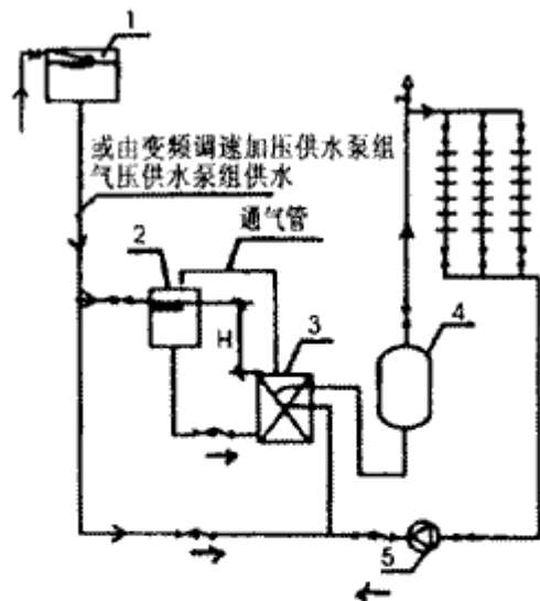
图 3 间接加热热水机组配贮热水罐热水供应系统 1-高位冷水箱;2-冷水补水箱; 3-机组;4-贮热水罐; 5-系统循环泵
