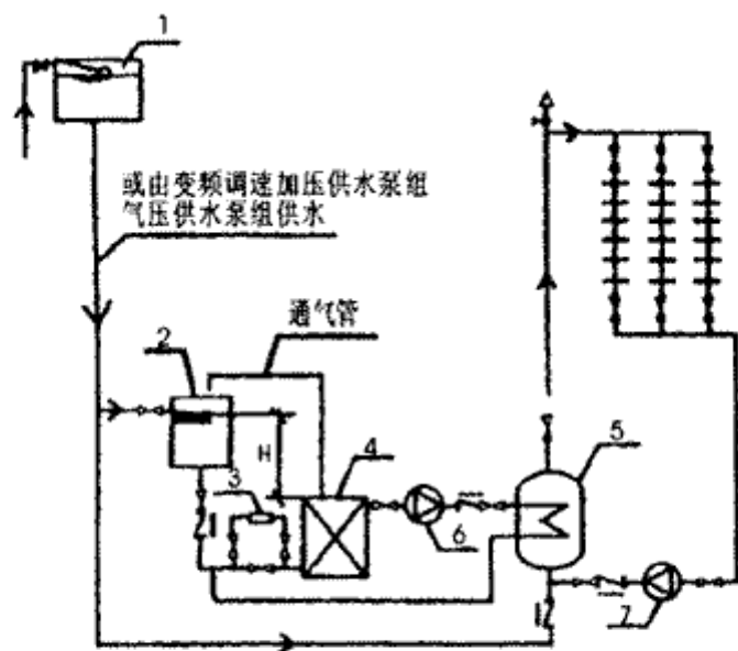
图 4 间接加热热水机组配容积式或半容积式水加热器的热水供应系统 1-高位冷水箱;2-冷水补水箱;3-水质稳定或软化处理装置;4-机组; 5-导流型容积式或半容积式水加热器;6-热媒循环泵;7-系统循环泵
