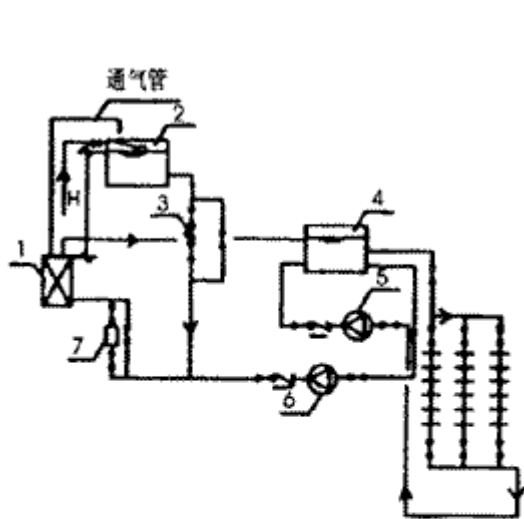
图 2 屋顶层设置机组热水供应系统 1-机组;2-冷水箱;3-电磁阀; 4-热水贮水箱;5-系统循环泵; 6-热媒循环泵; 7-软化处理或水质稳定处理装置
