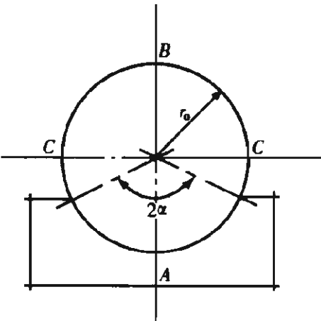
图 D. 0. 2-1 混凝土基础计算图
