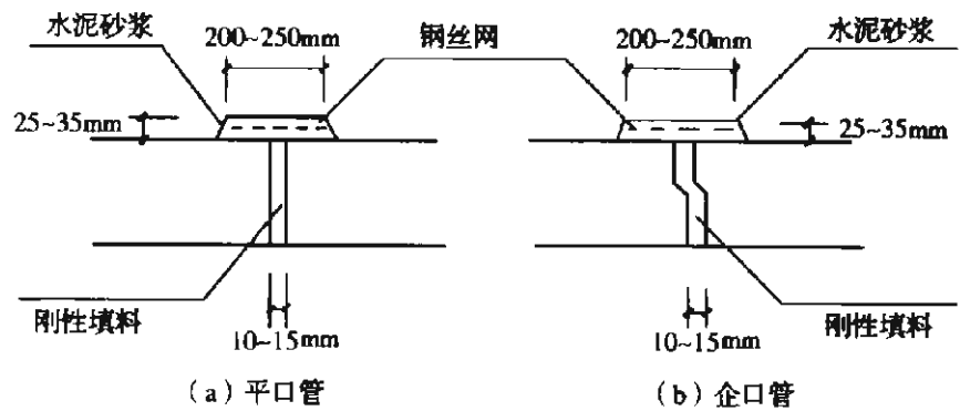
图 7.2.1 钢丝网水泥抹带接口
