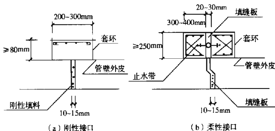
7.3.1 现浇套环接口
