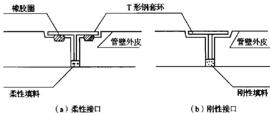
图 7.6.1 双插口管接口
