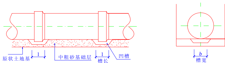
图 6.3.3 管道接口处的凹槽
