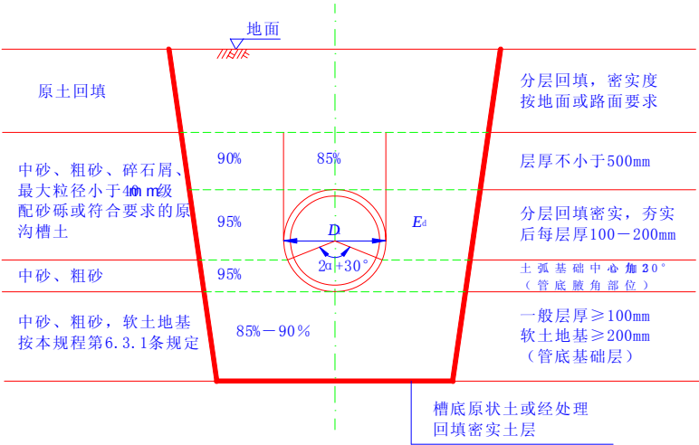
图 8.2.5 沟槽回填土要求
