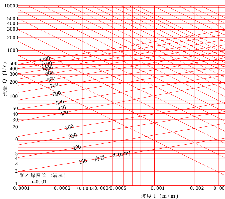
图 A. 0.1 满流条件下聚乙烯管管道水力计算图(内径 15
