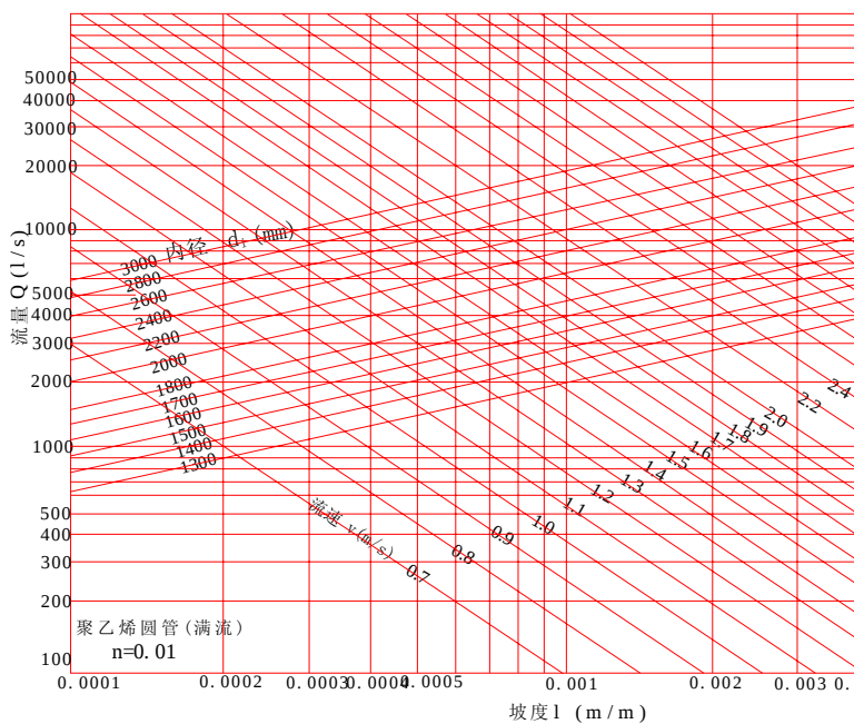
图 A.0.2 满流条件下聚乙烯管管道水力计算图(内径 13
