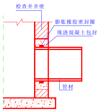
图7.0.2 现浇混凝土包封连接 图7.0.3 管道与检查井预留洞的连接
