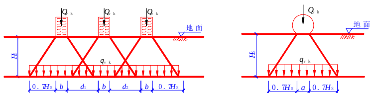
(a)顺轮胎着地宽度方向的压力分布 (b)顺轮胎着地长度方向的压力分布
