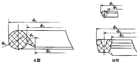
图 3.0.7 橡胶密封圈
