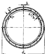
图 3.0.2 中空壁消音硬聚氯乙烯螺旋管剖面
