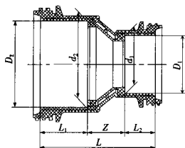
图 A.0.7 异径管箍
