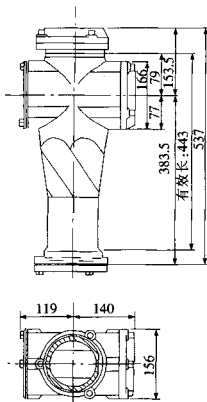
图 B.1.2 三通旋流器
