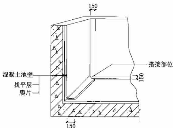
图 5.2.9 泳池阴角三角交接部位节点的构造
