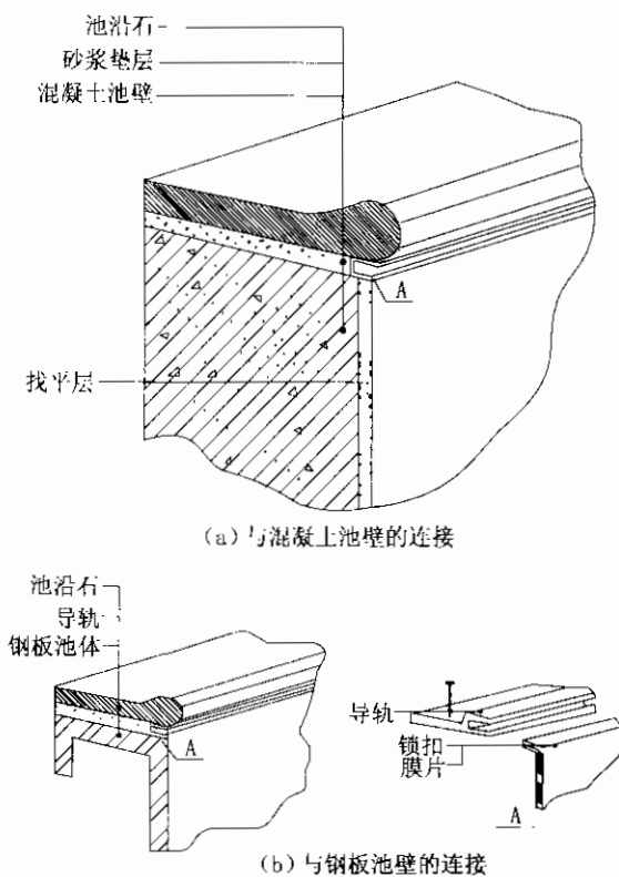
图 5.2.4 膜片平导轨连接节点的构造
