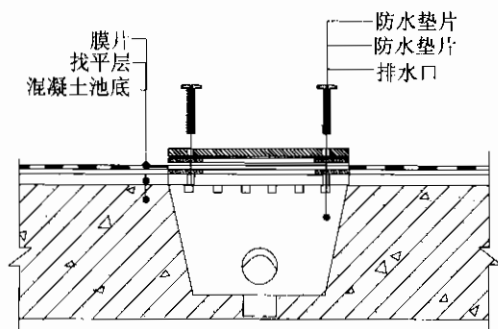
图 5.2.11 排水口节点
