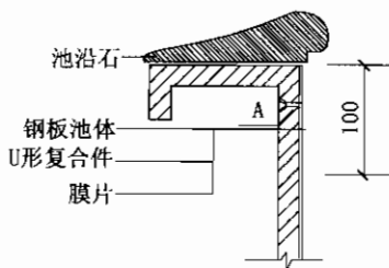
(b) 与钢板池壁的连接
