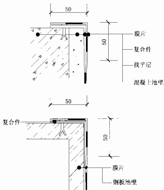
图 5.2.2 L 型钢复合件连接节点的构造
