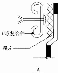
图 5.2.3 U 形型钢复合件连接节点的构造
