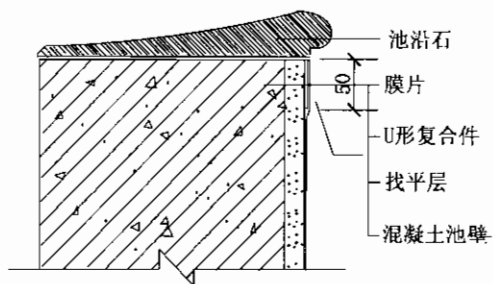
(a) 与混凝土池壁的连接
