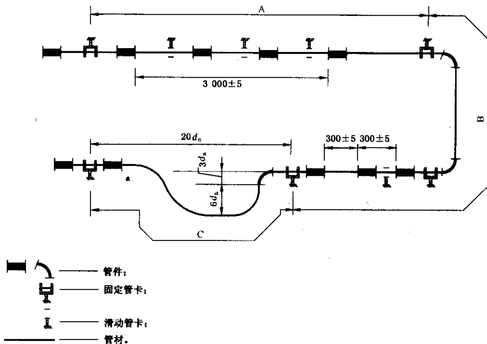
图 A.1 试验安装
