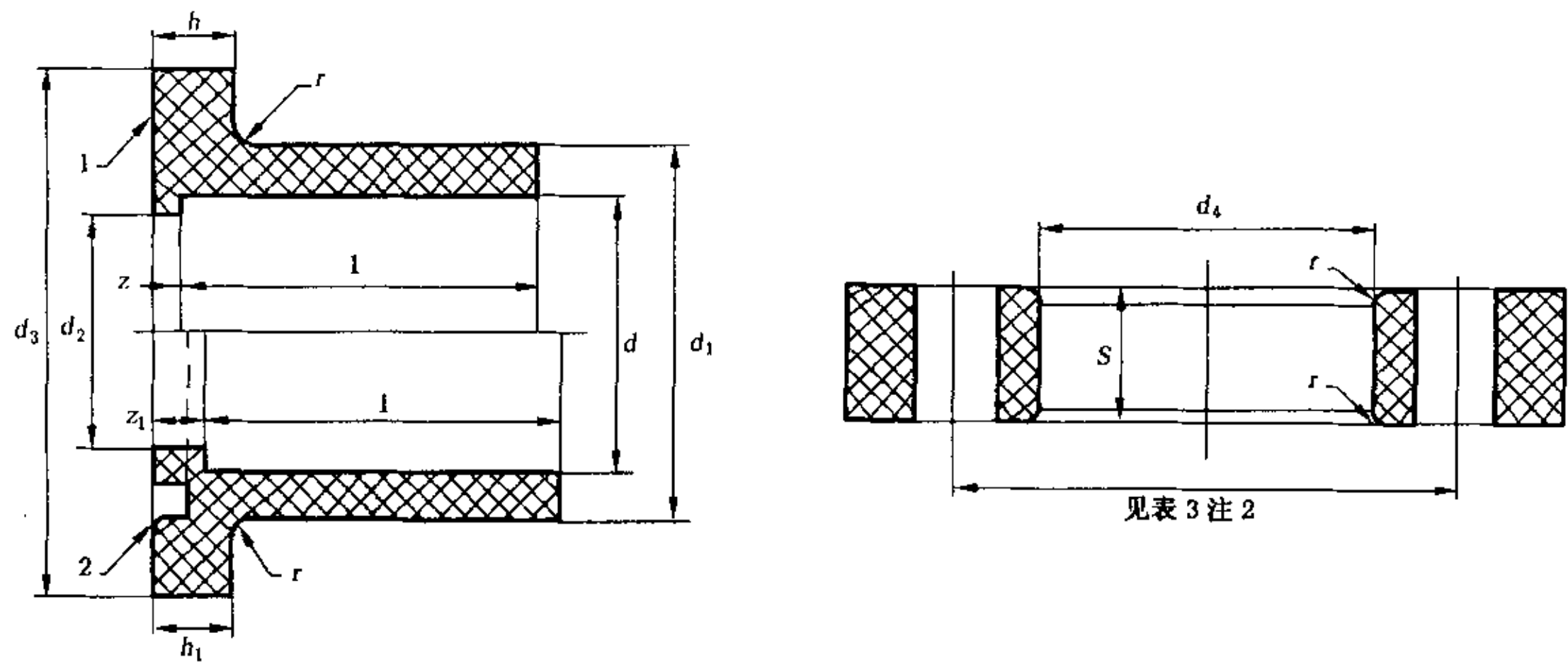
1——平面垫圈接合面； 2——密封圈槽接合面。
