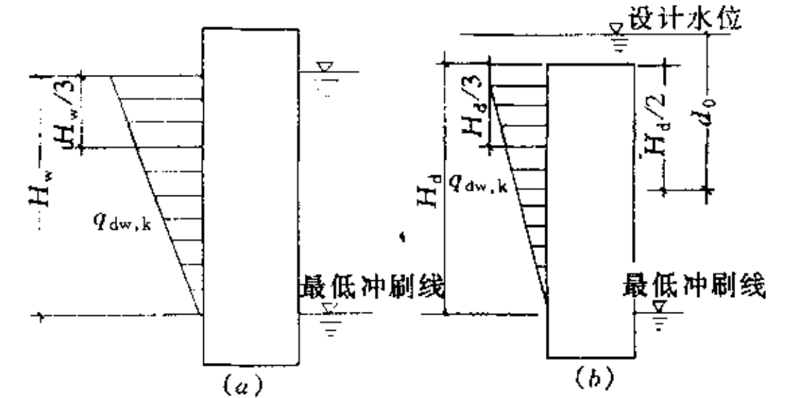
图 4.3.4 作用在取水头部上的流水压力图 (a) 非淹没式；(b) 淹没式
