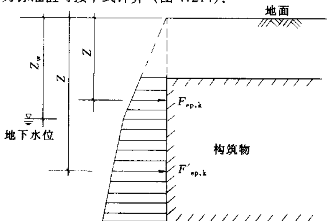
图 4.2.4 侧壁上的主动土压力分布图
