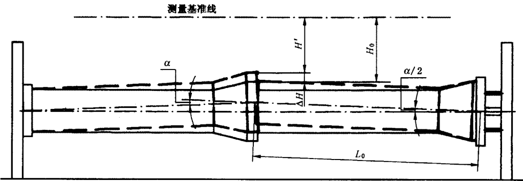
图 8 管子转角接头密封性能试验示意图
