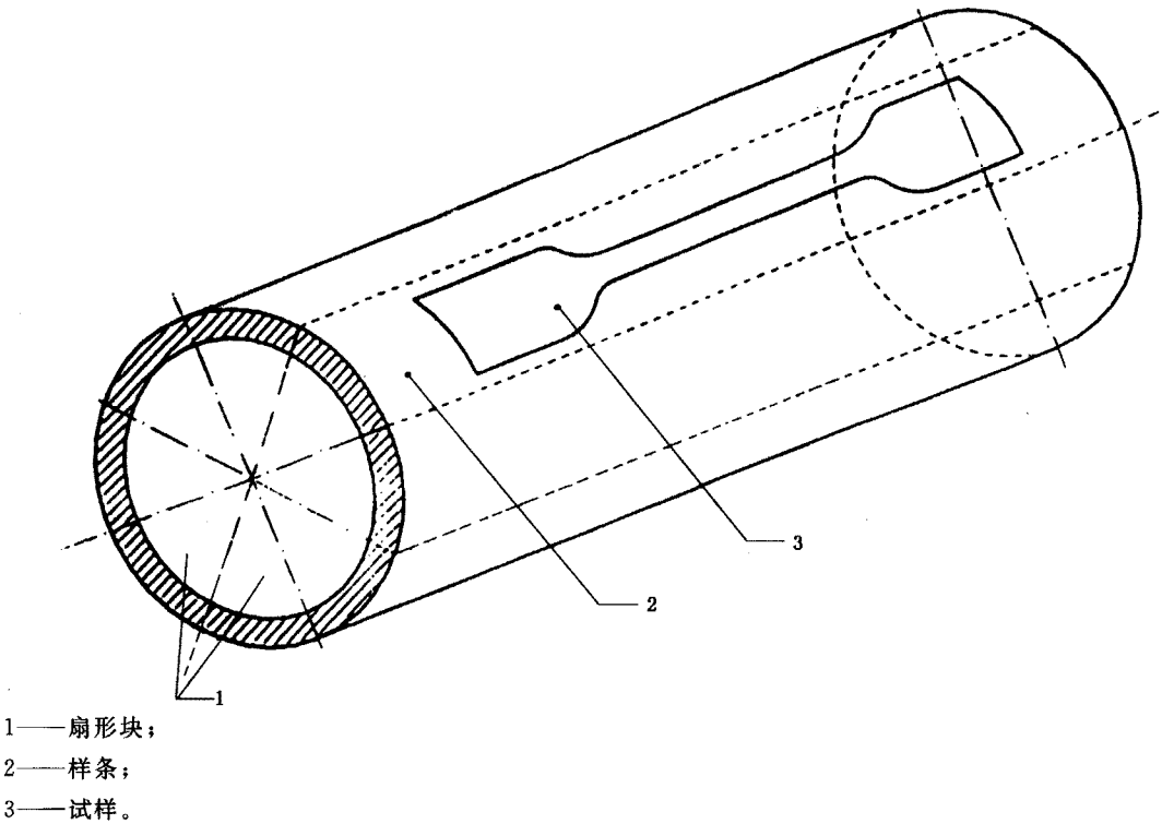
图 1 试样制备
