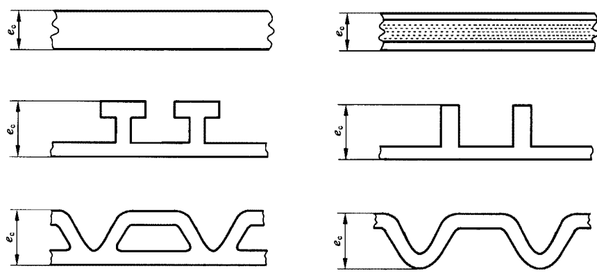
图 4 管壁厚度 e_c 示例
