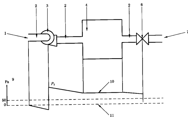
图 C.1 b) 保护气体排气口具有火花和颗粒隔板
