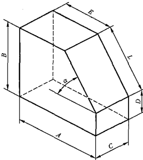
图 6 拱脚砖
