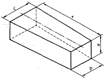
图 5 竖宽楔形砖
