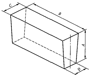
图3 侧厚楔形砖
