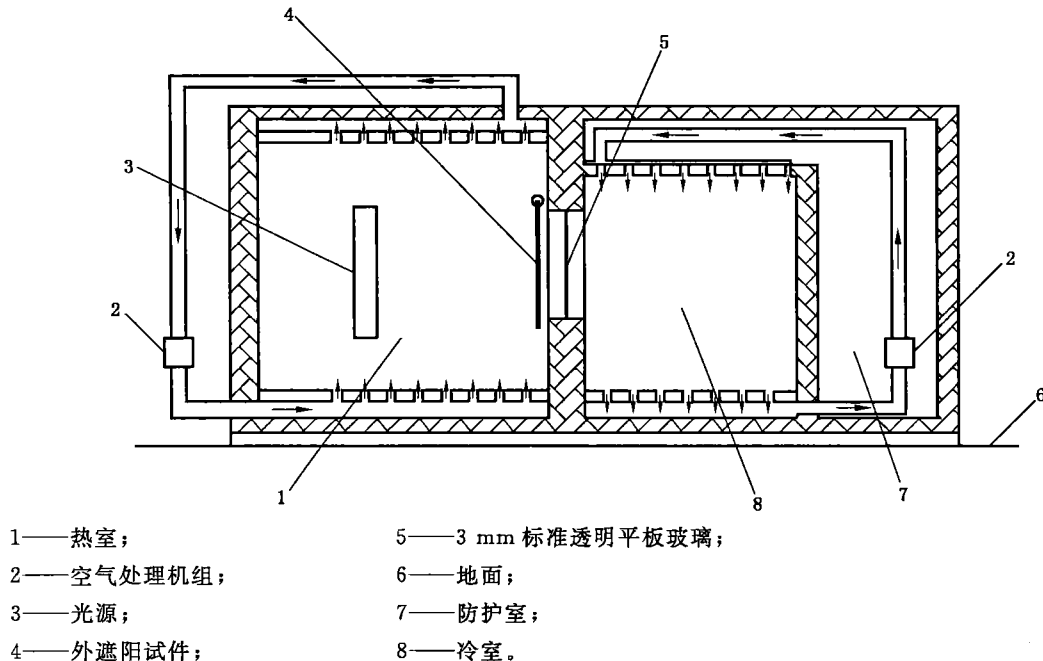
图 1 人工光源法试验装置示意图
