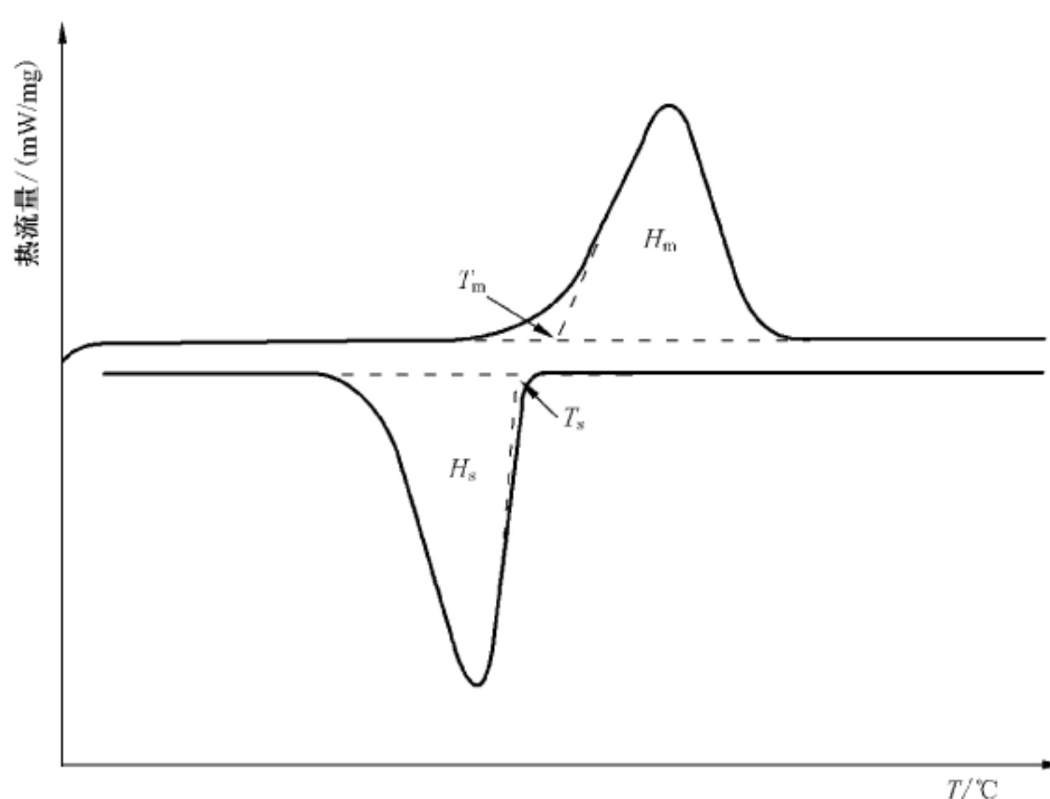
图 3 典型相变材料 DSC 测试曲线
