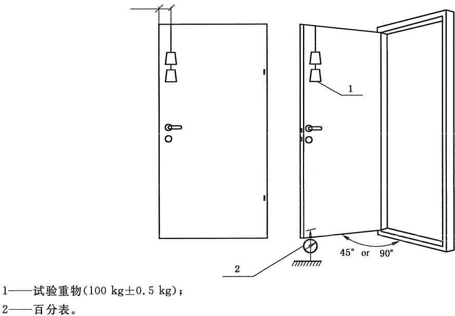
图 4 悬端吊重试验
