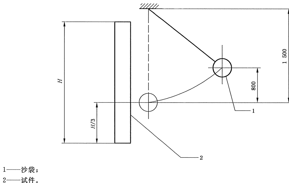
图 3 软冲击试验
