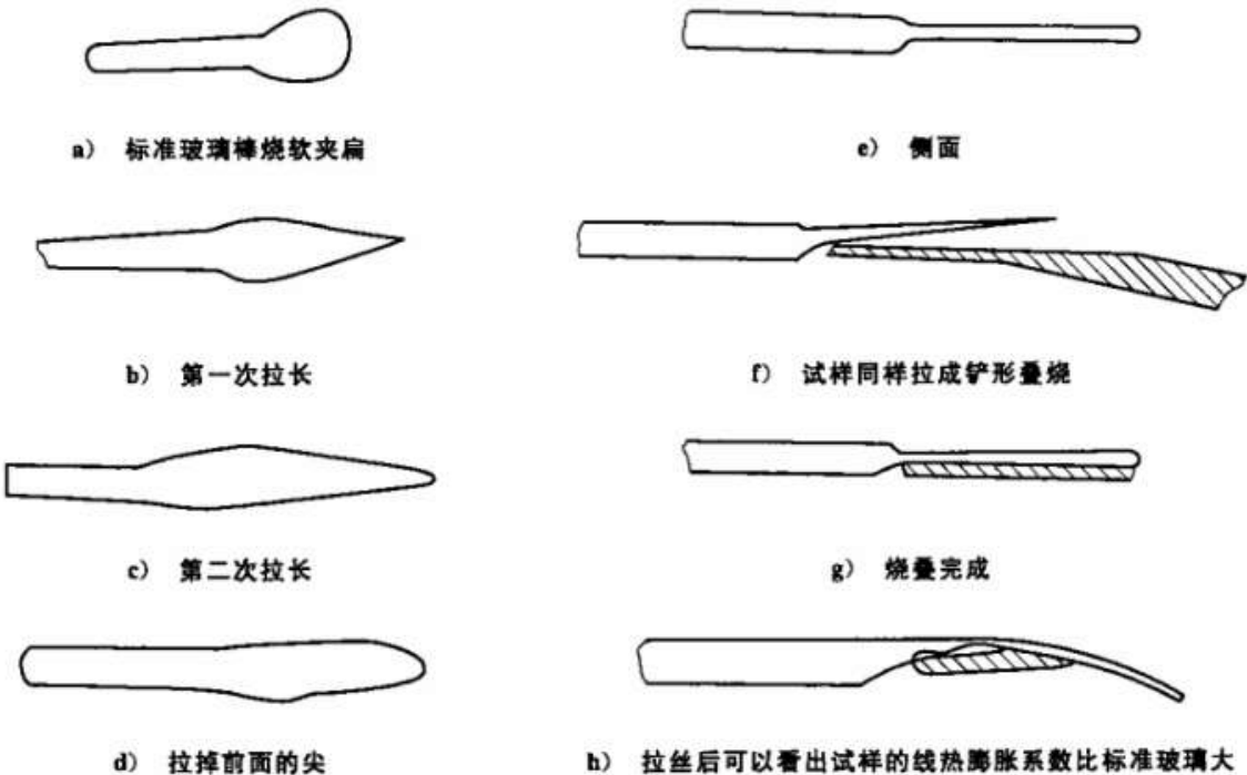
图 3 拉丝过程
