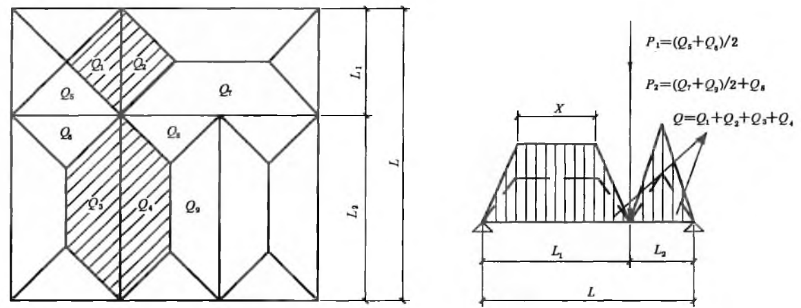
说明： L_1 ——集中荷载受力点到杆件较远一端的长度，单位为毫米(mm)； L_2 ——集中荷载受力点到杆件较近一端的长度，单位为毫米(mm)； P_1, P_2 \dots P_n ——由其他受力杆件传递的集中荷载，单位为牛顿(N)； X ——为梯形荷载的顶宽，单位为毫米(mm)。
