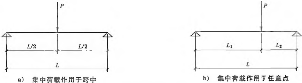
图 B.9 简支梁承受集中荷载示意图
