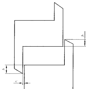
图 1 上悬窗、平开窗、下悬窗、平开下悬窗、中悬窗
