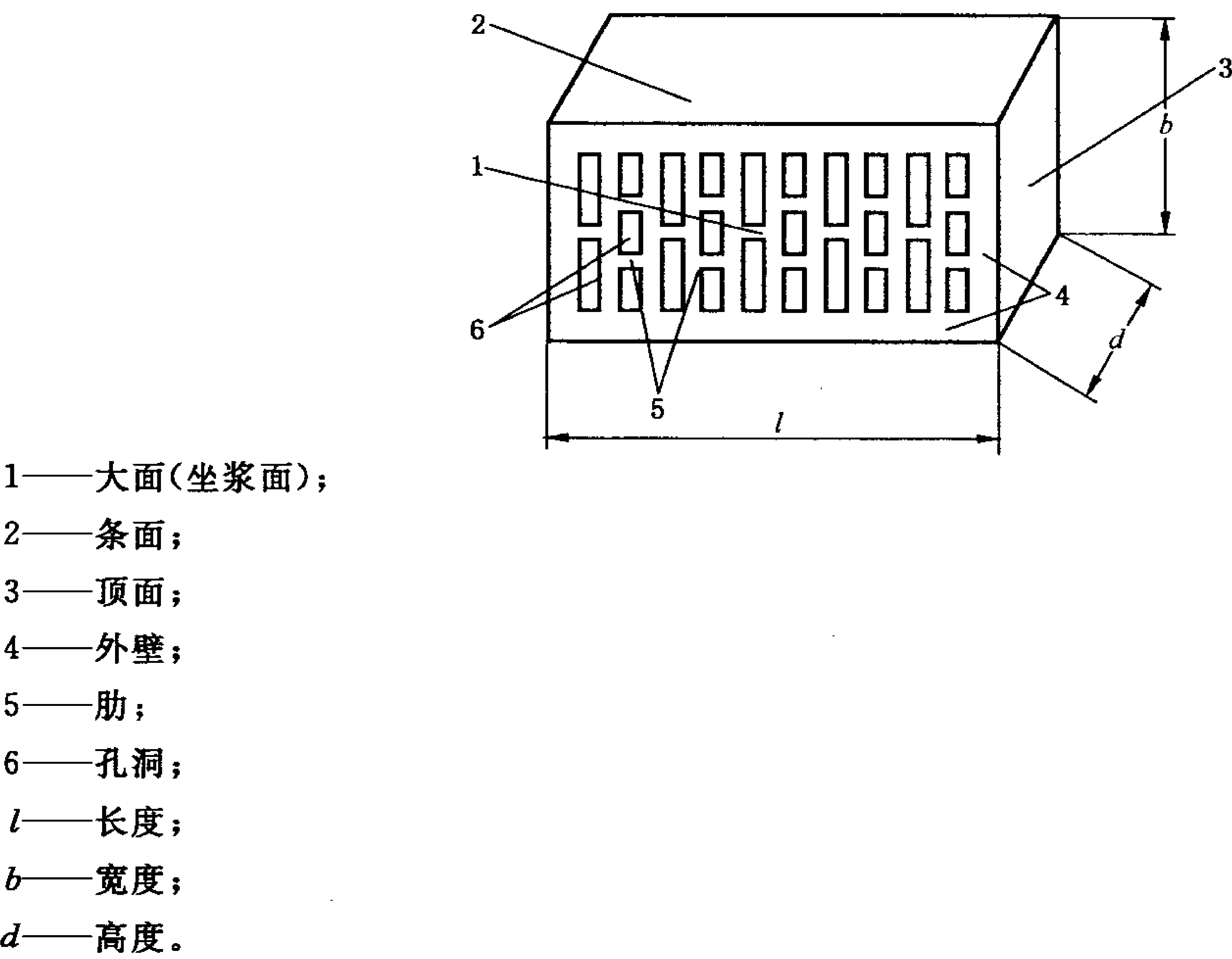
图 B.1 砖各部位名称
