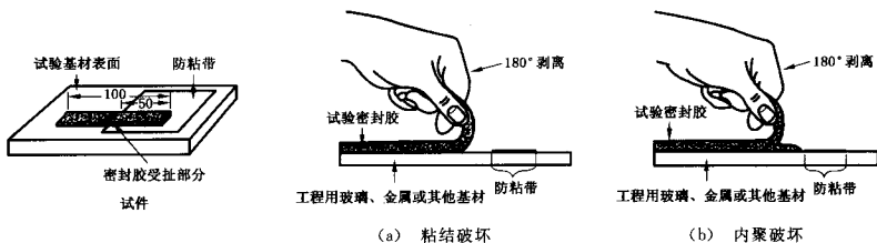
图 D.2 非破坏手拉剥离试验
