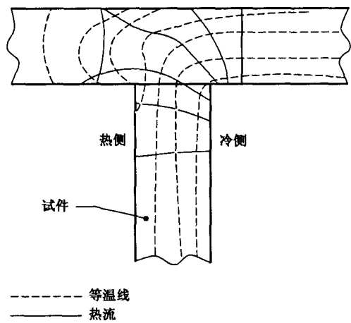
图 3 试件和框架中热流路径
