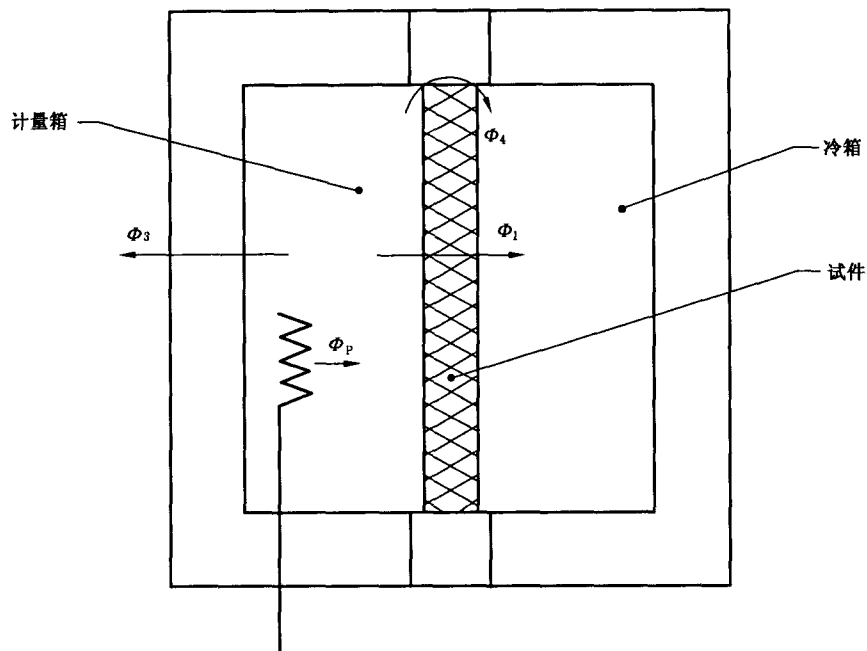
图 2 标定热箱
