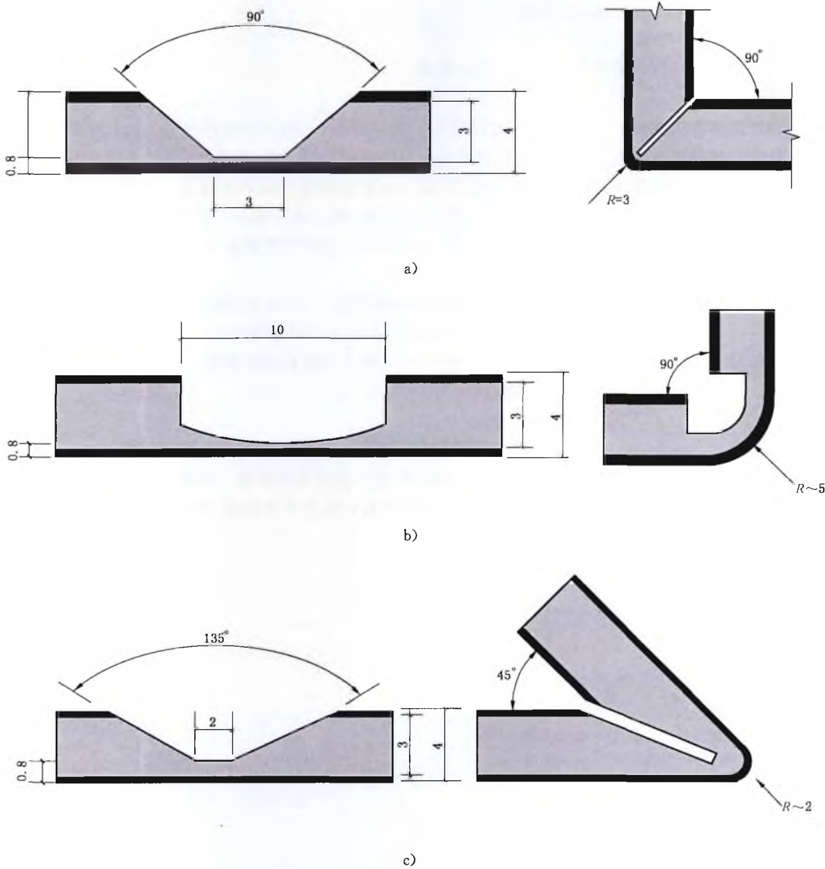
图 C.1 几种典型的加工开槽示意图
