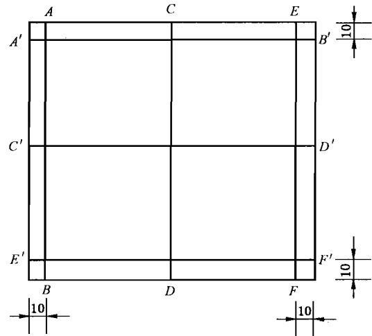
图 6 热膨胀系数测量位置示意图
