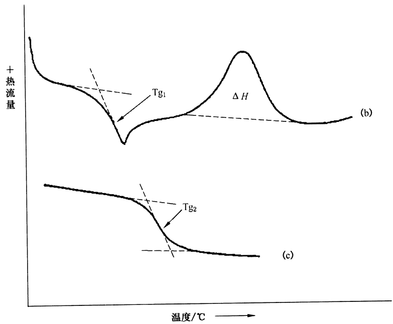
图 B.1 对环氧粉末热扫描
