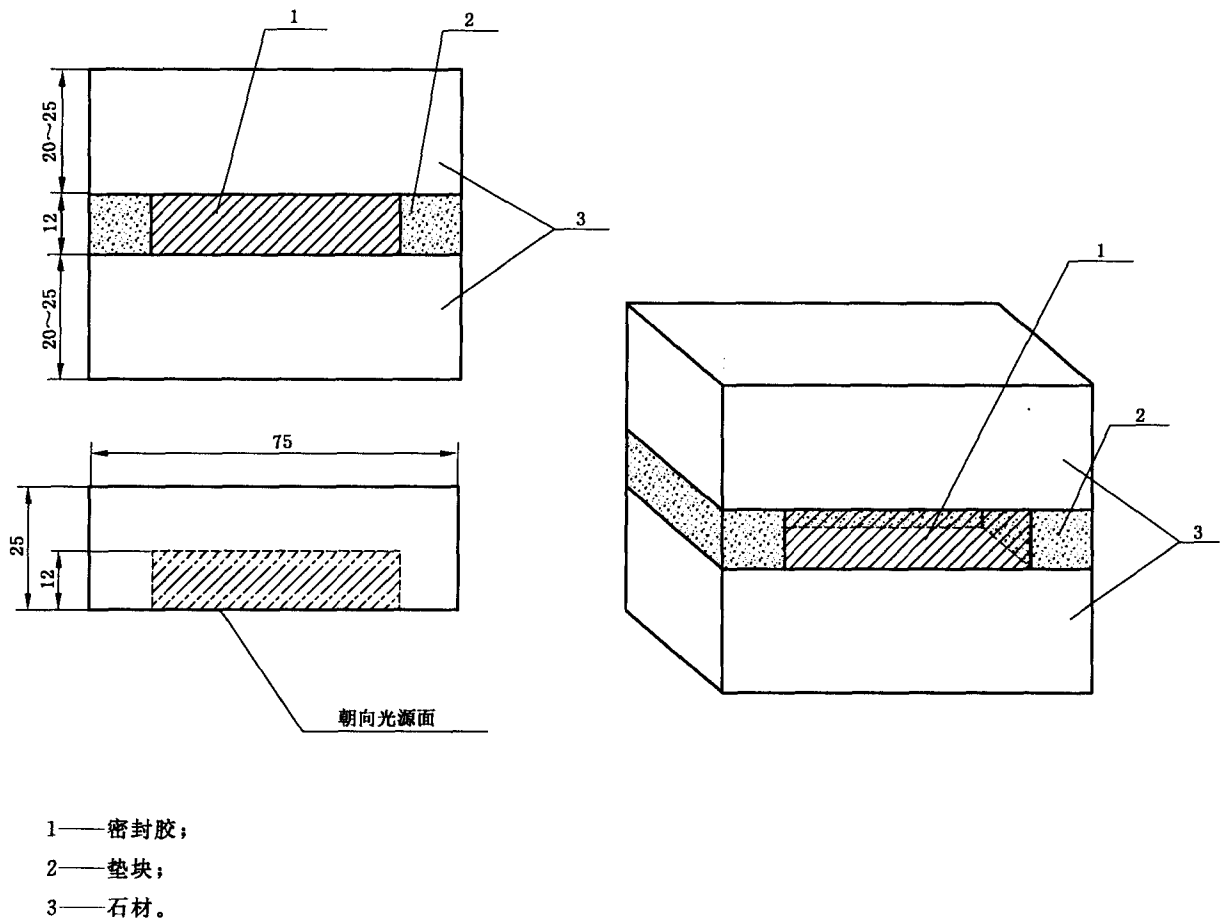
图 1 试件形状
