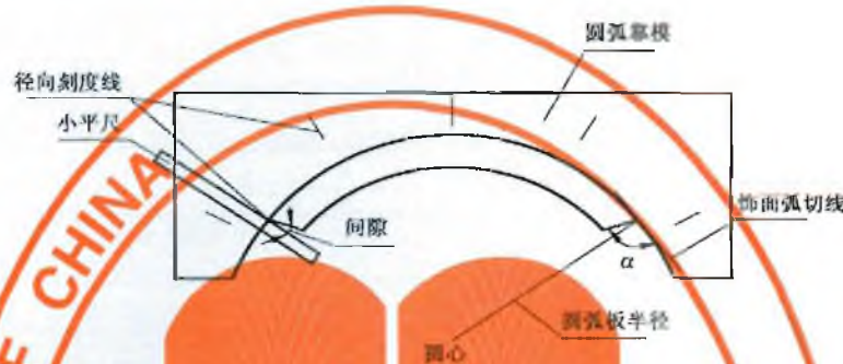
图 5 侧面角测量
