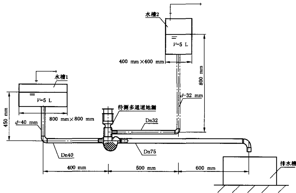
图 B.5 多通道地漏自清能力试验装置
