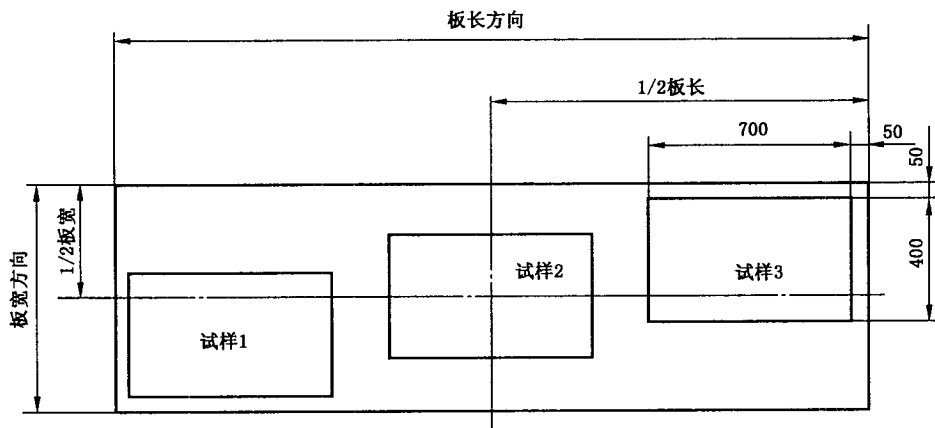
图 1 试样在样本中的分布示意图
