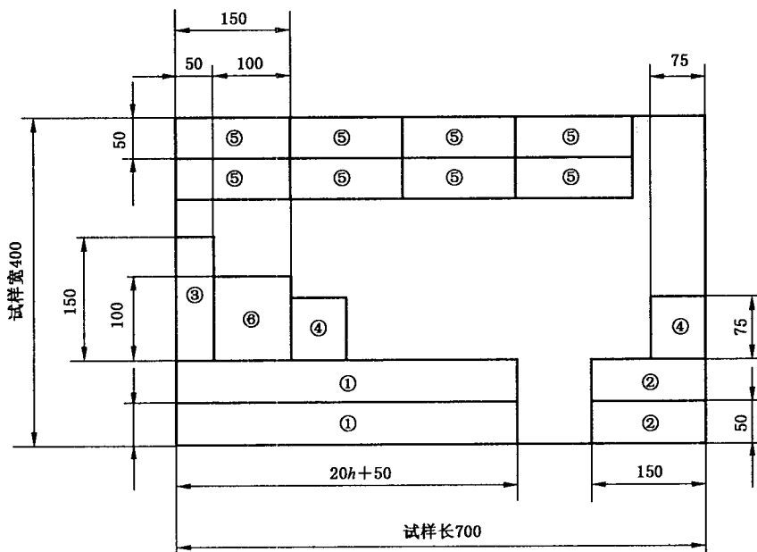
图 2 试件的配置示意图
