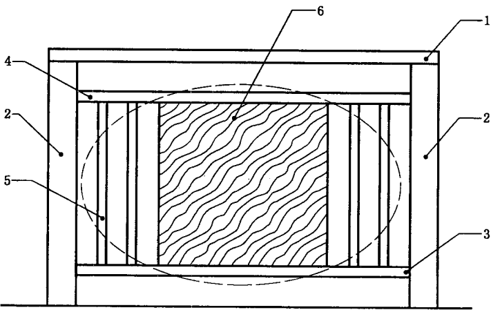
图 1 护栏体系的典型结构图
