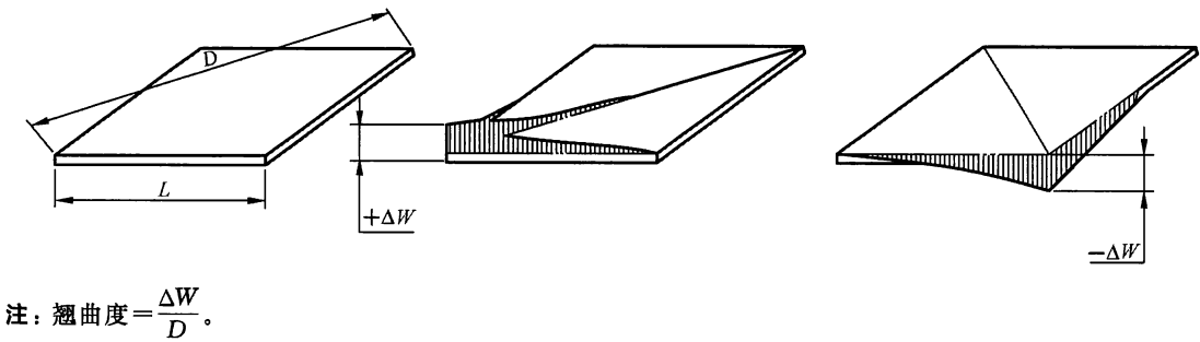
图 5 翘曲度
