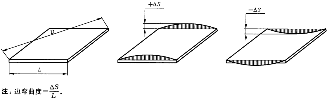
图 4 边弯曲度
