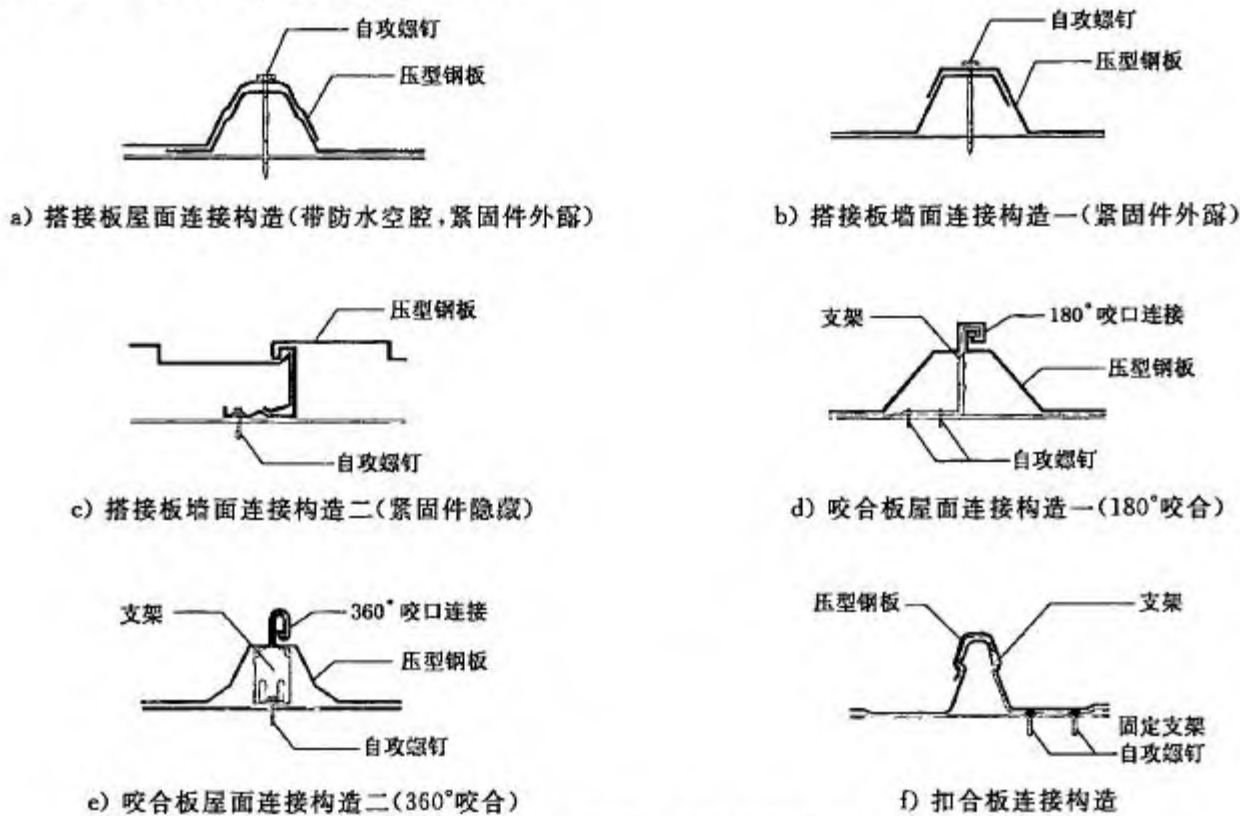
图 2 压型钢板典型连接构造
