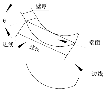
图3 曲面板的弦长、高度、壁厚等
