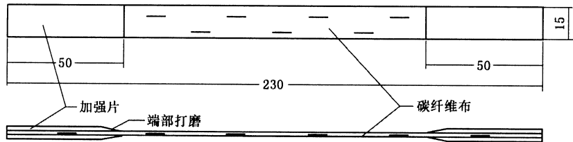
图 A.1 碳纤维布试样外观尺寸
