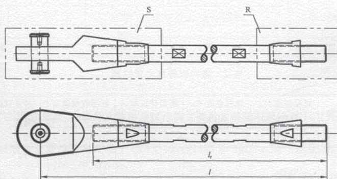
图 5 DR 型钢质拉杆构件
