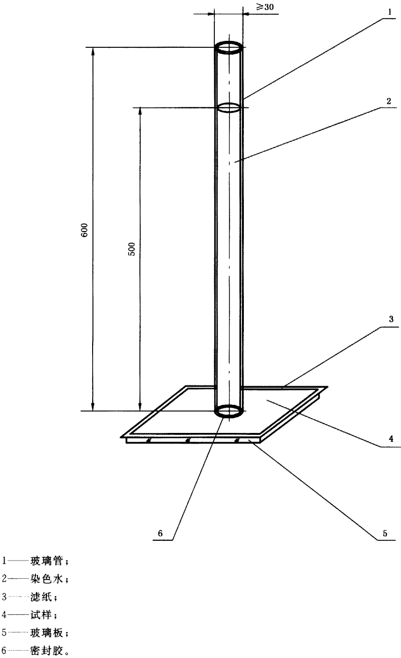
图 5 穿孔水密性试验装置
