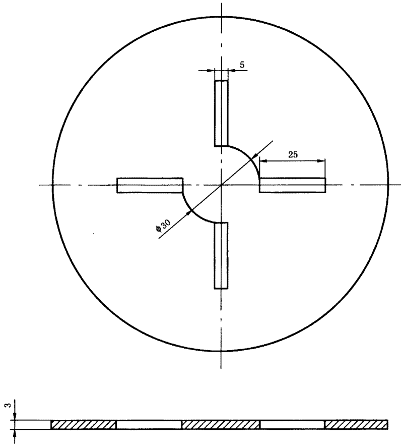
图 6 金属开缝槽盘
